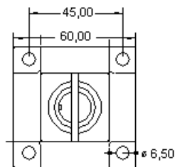
Aufschraubflansch
